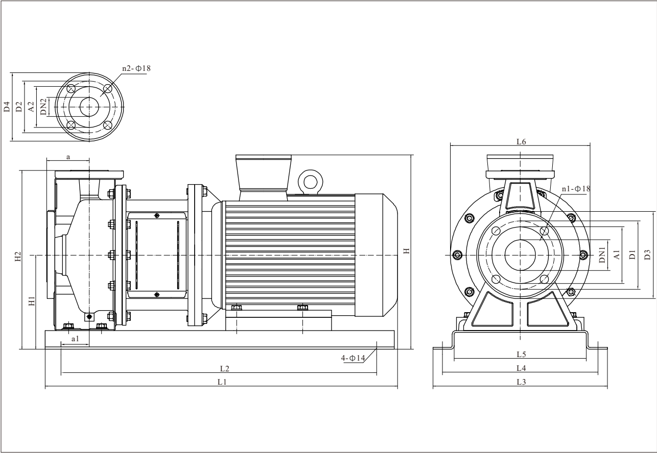
安装图
