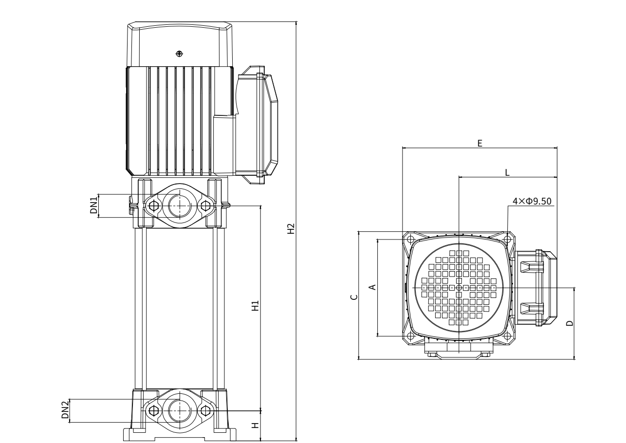
外形尺寸图 Overall Dimension
