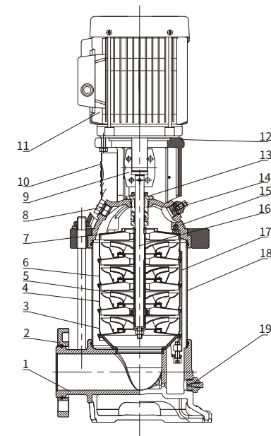
泵结构图 Structure Diagram
