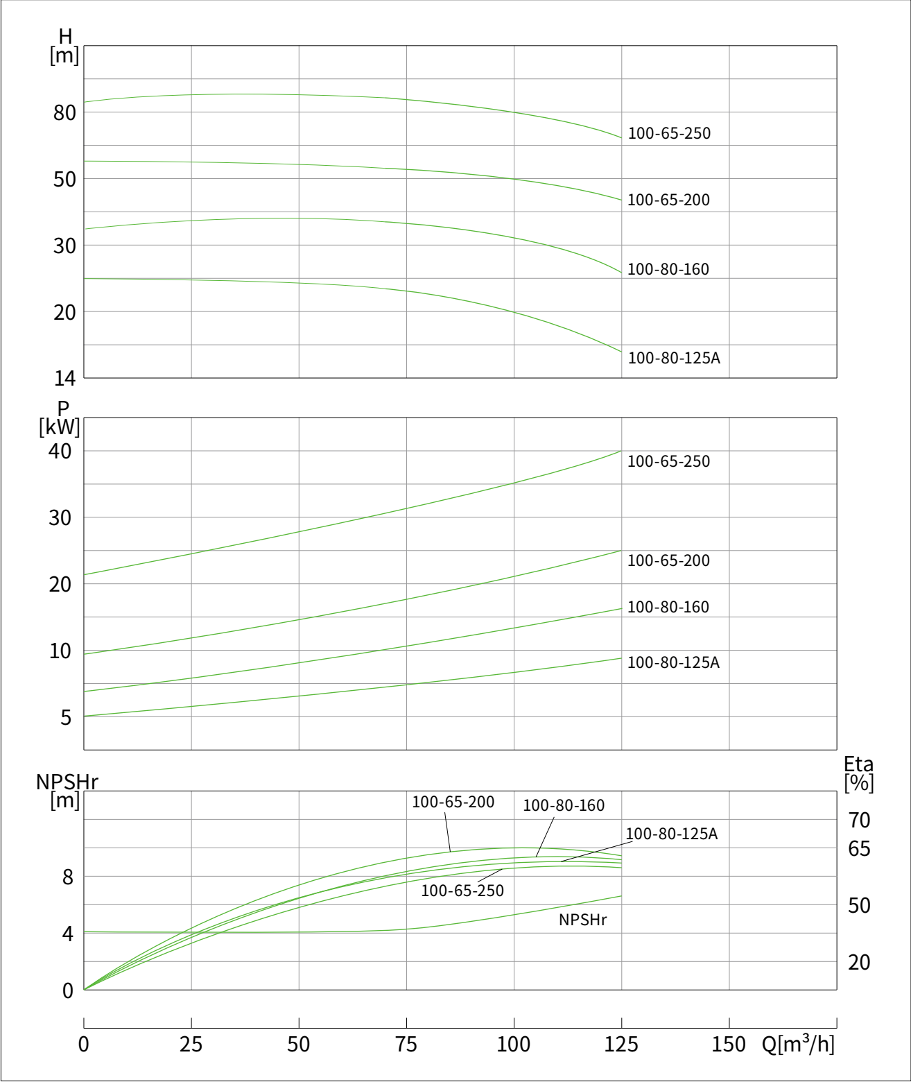
性能曲线 Performance Curves ASZ100
