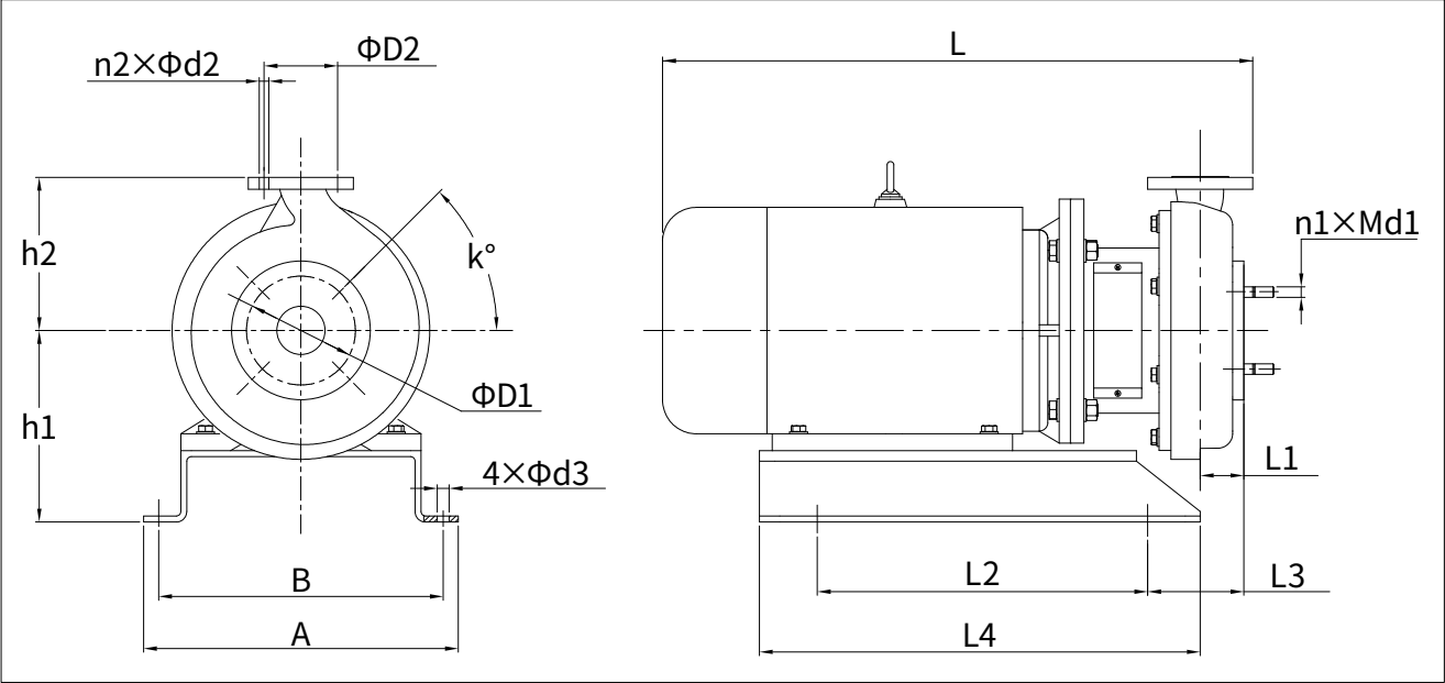
安装图 Installation Diagram
