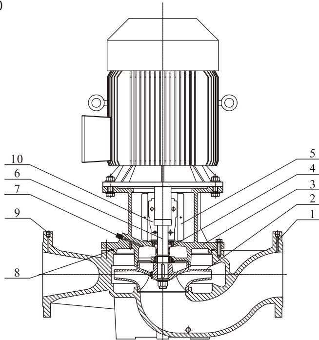
截面图 ALG200~ALG250
